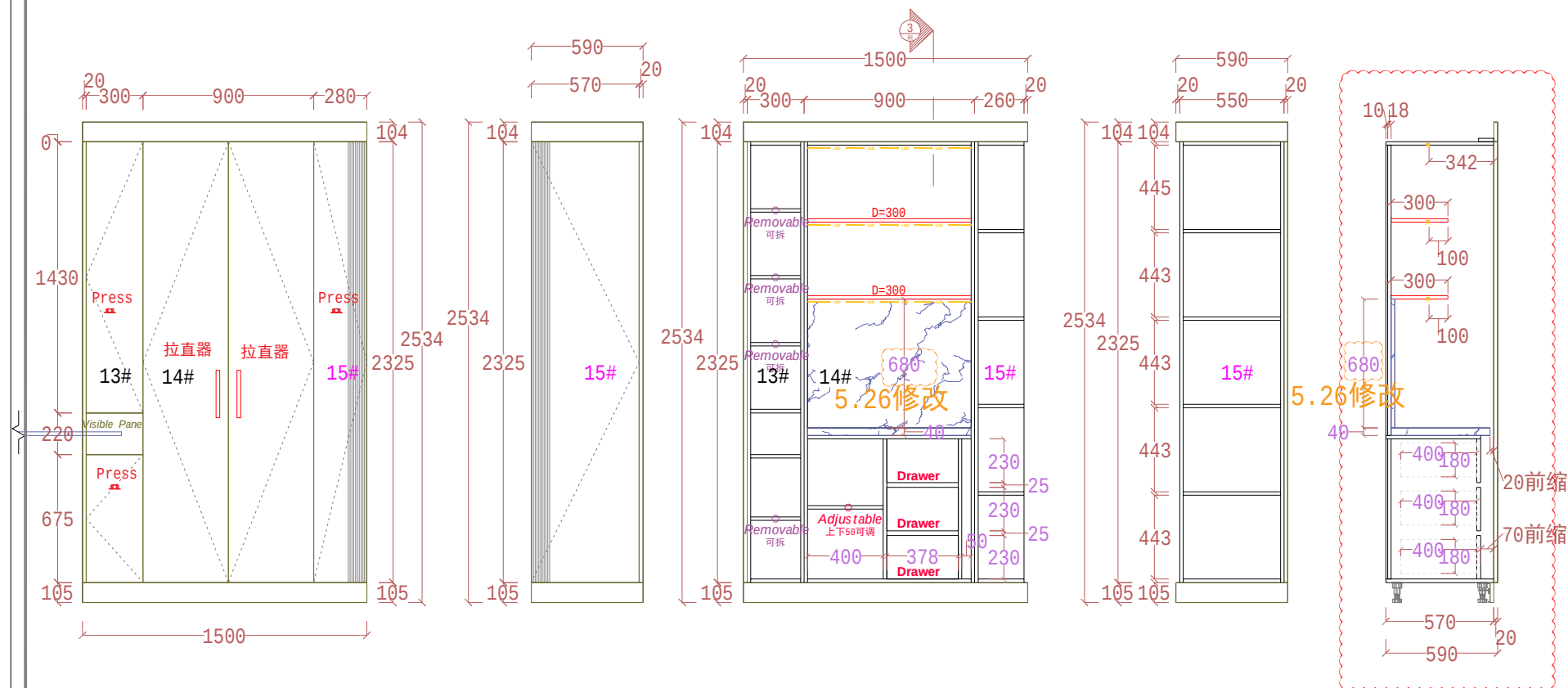
ELEVATION G
