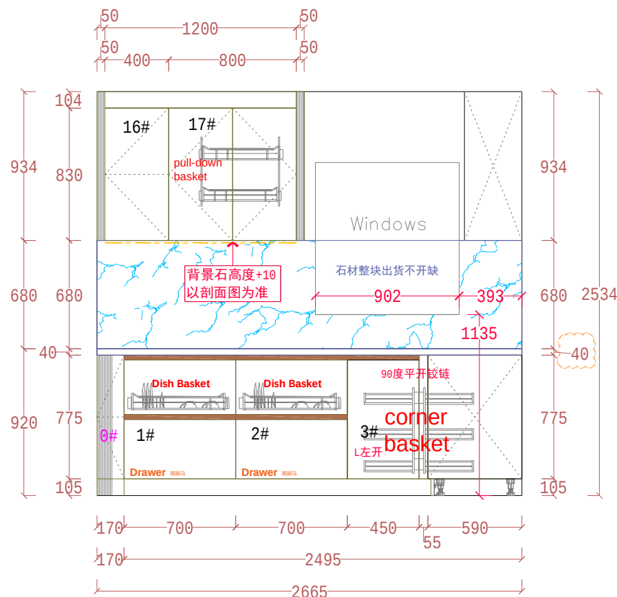
ELEVATION B
